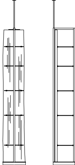
Modulo libreria/bookcase module L1920 - cm 42x39x249h
